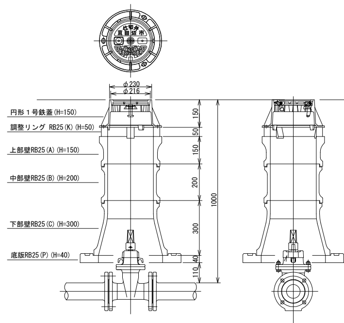
消火栓用 50型 H=1200mm
