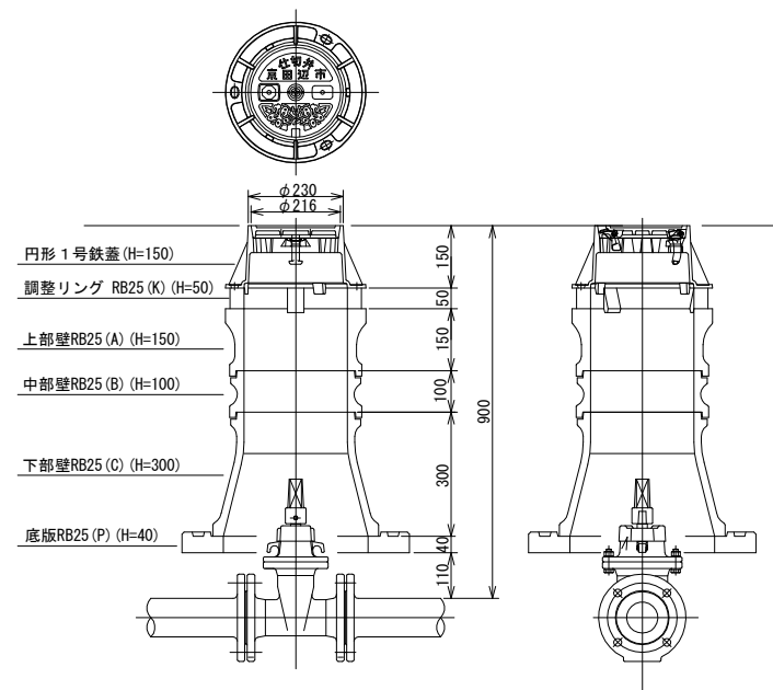
仕切弁用 25型 H=900mm
