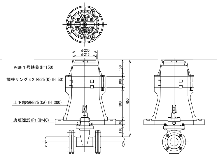
仕切弁用 25型 H=700mm
