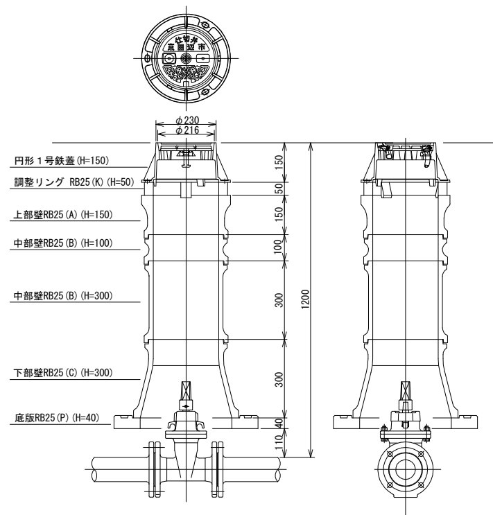
仕切弁用 25型 H=1200mm
