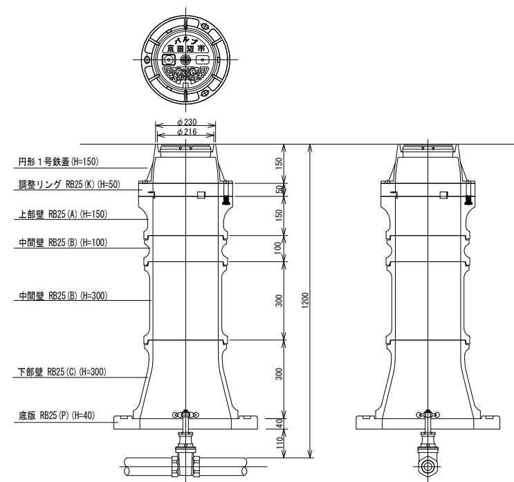
バルブ用 25型 H=1200mm
