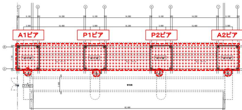
工事対象建物(既存全体平面図)
