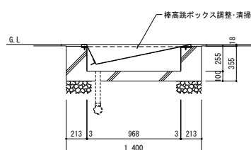
断面図
