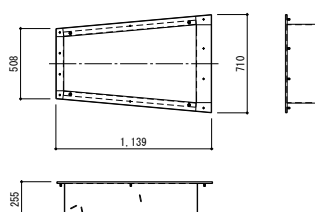
ボックス受枠 詳細図
