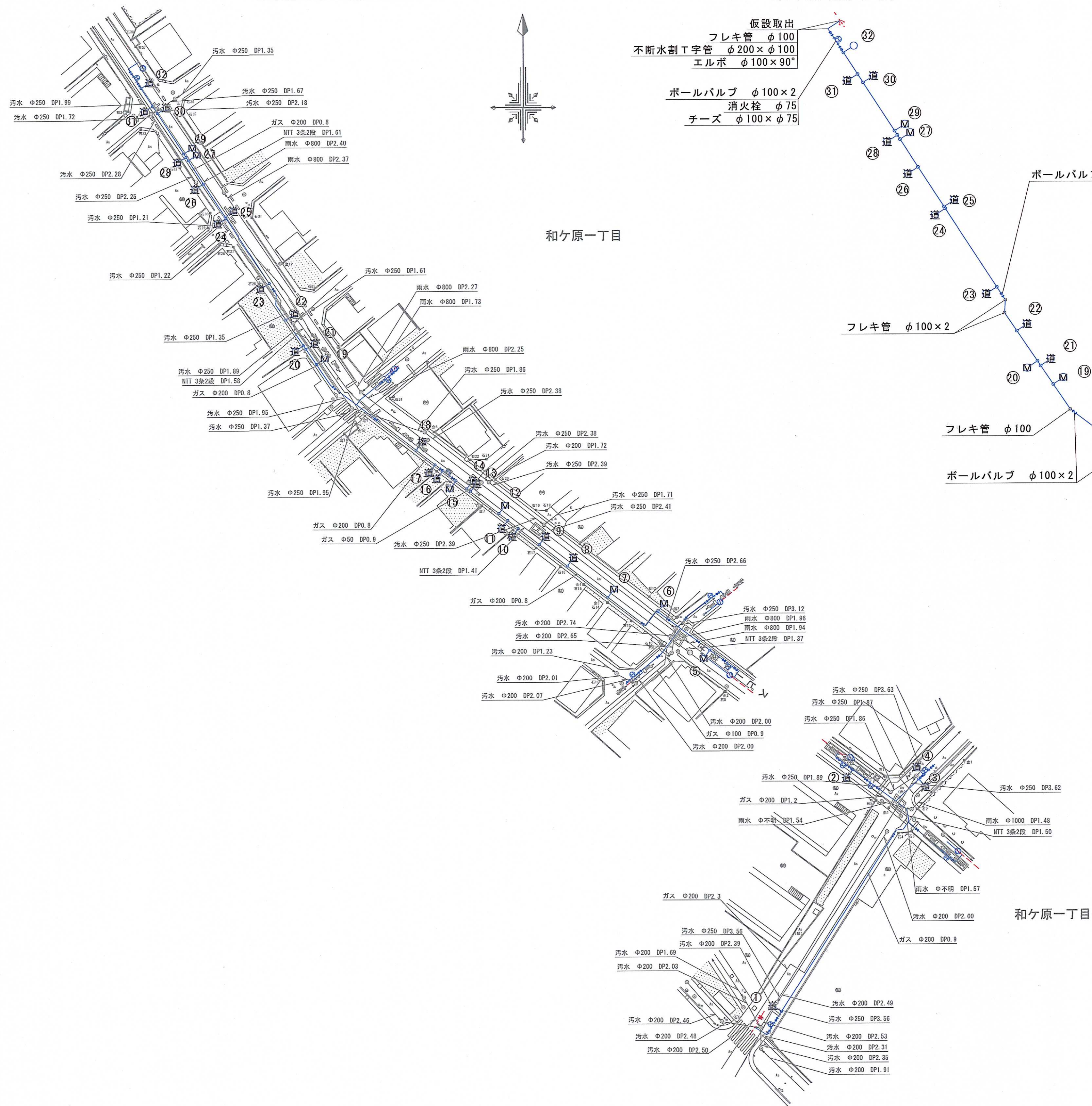
仮設平面図 1/500
