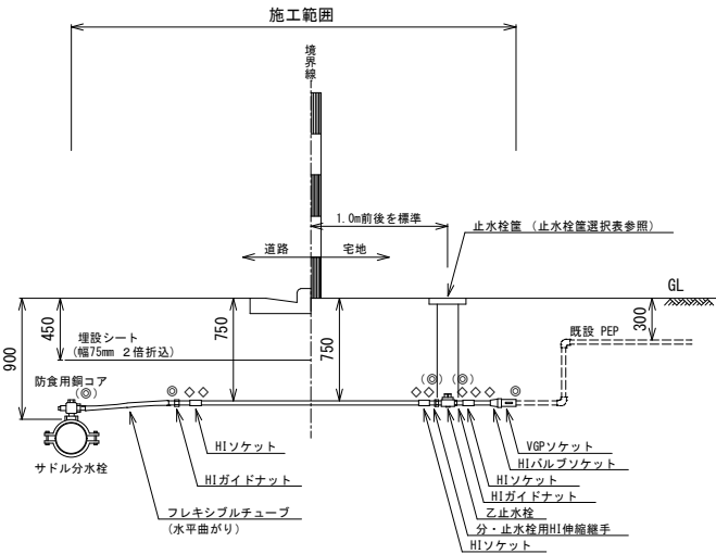
給水装置分岐替標準図
