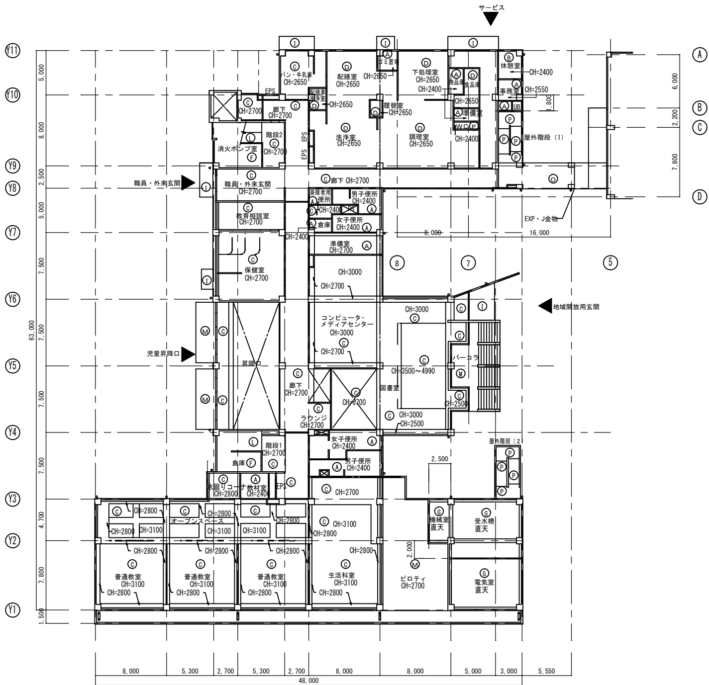
1階天井伏図
