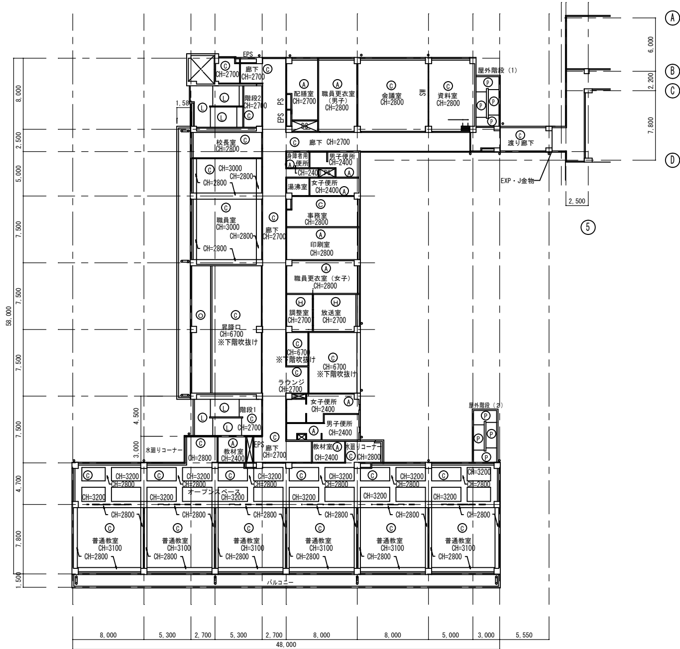
2階天井伏図
