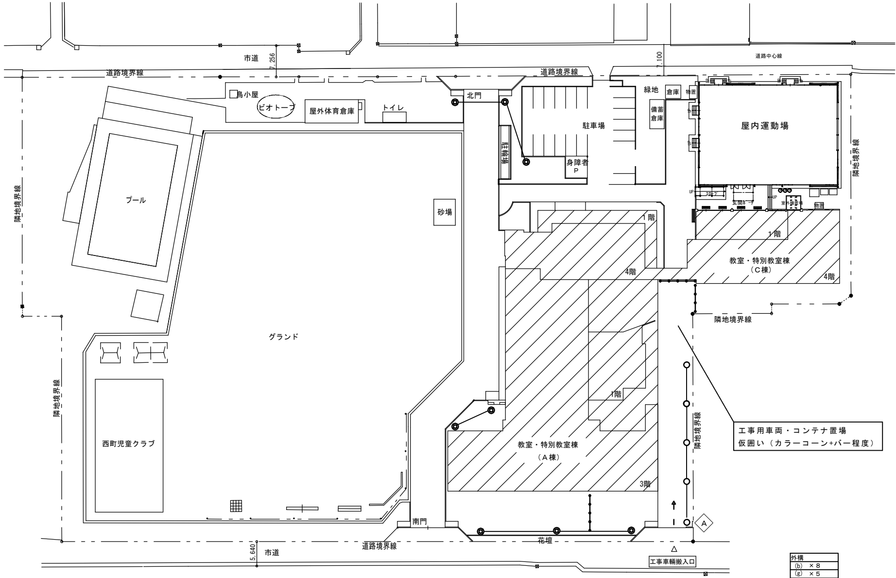
配置図・仮設計画図（参考図） S=1:600
