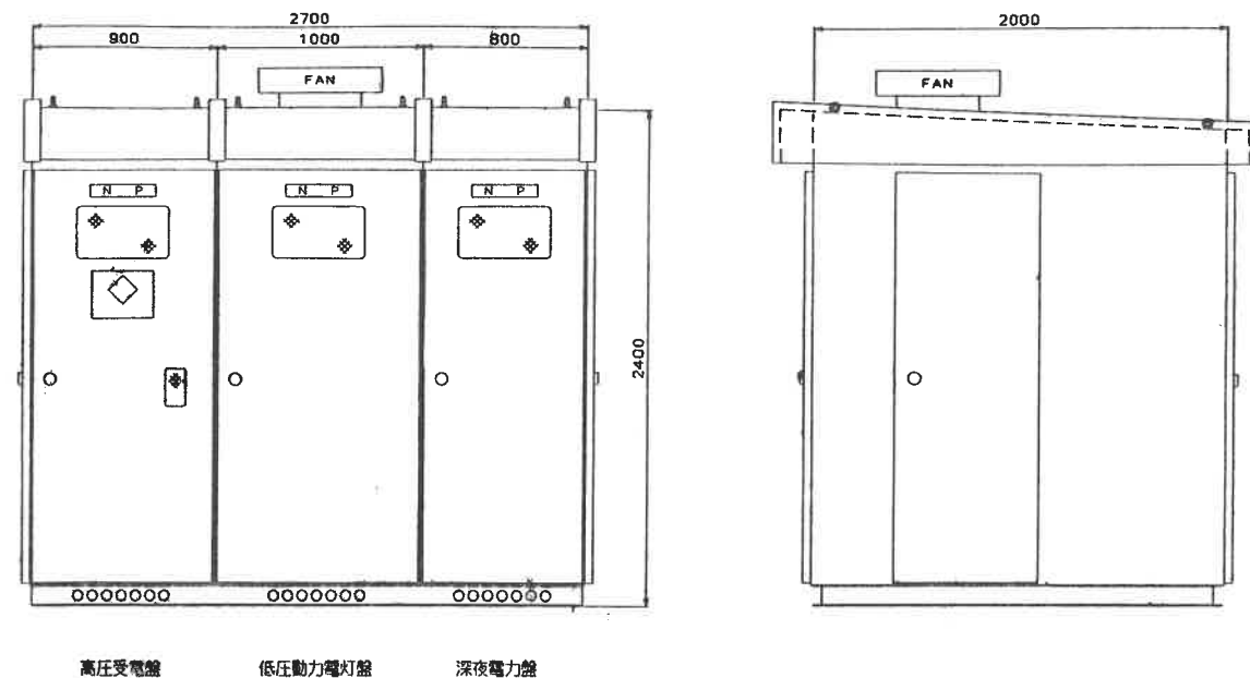
屋外キュービクル式受変電設備外形図 (参考)
