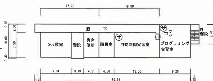
2階 平面図
