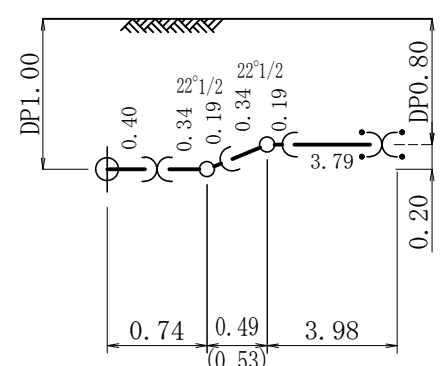
② - ②' 詳細図
