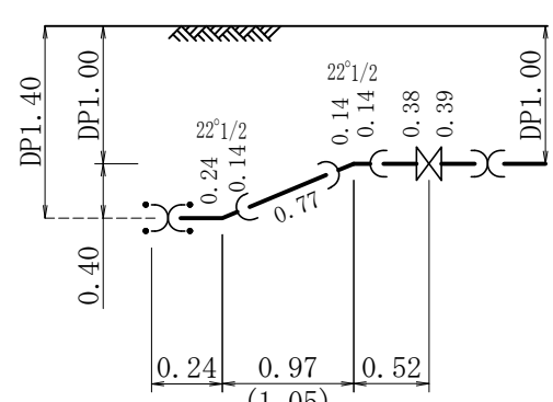
③ - ③' 詳細図
