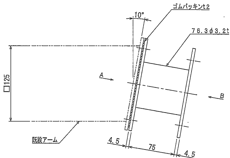
A矢視図
