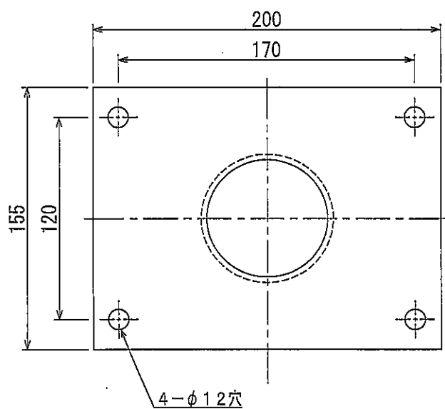
既設側プレート詳細
