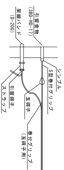
専用柱ケーブル引留図(コンクリート柱)
