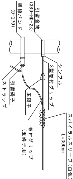
共架柱ケーブル引留図
