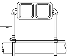
歩行者用灯器取付図
