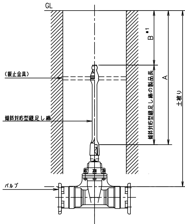
継足し棒組み合わせ表 DIP各種 ソフトシール弁
