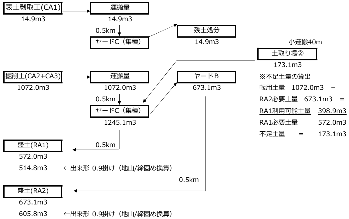
見込み土量収支
