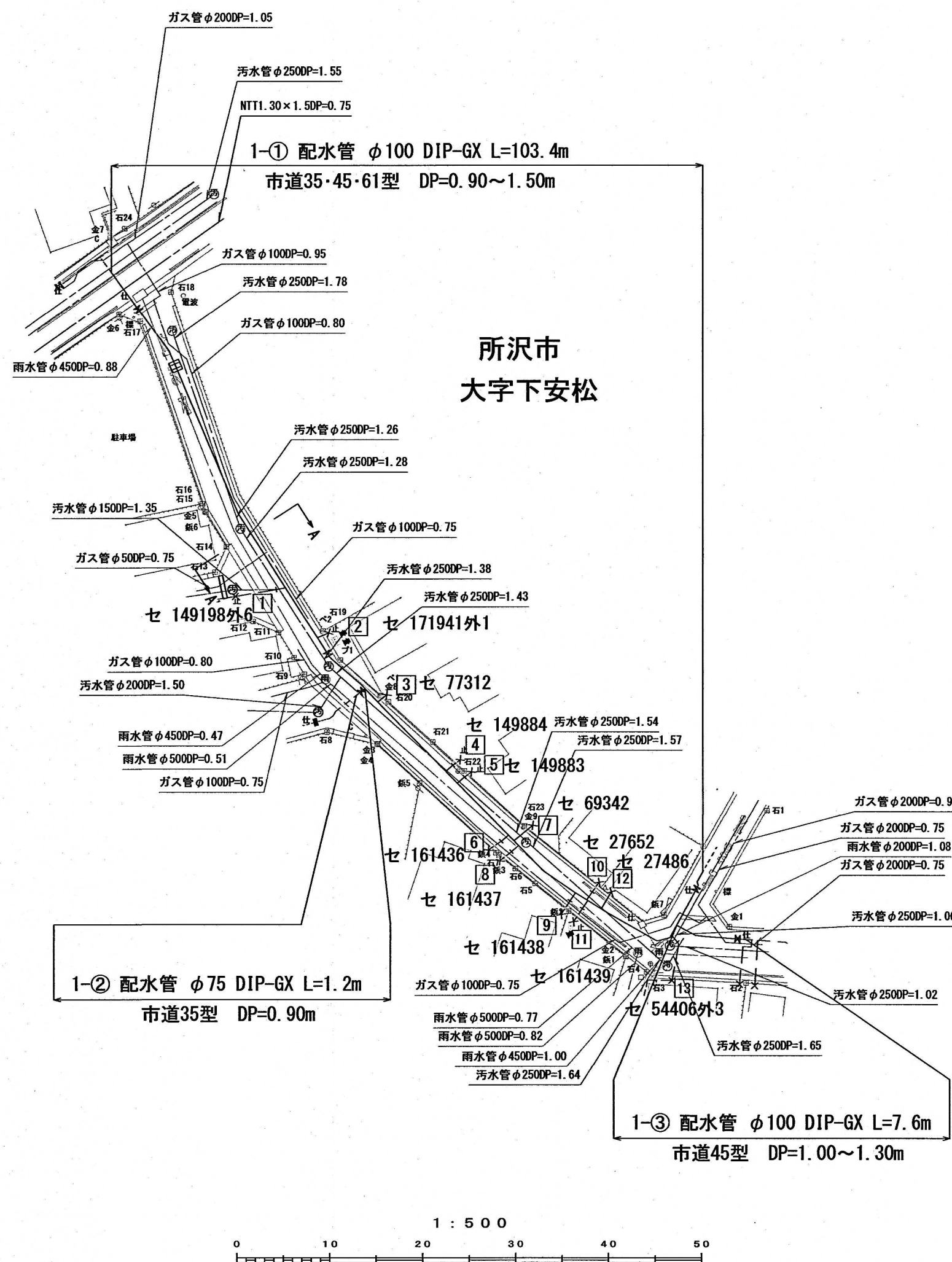
平面図 S=1/500
