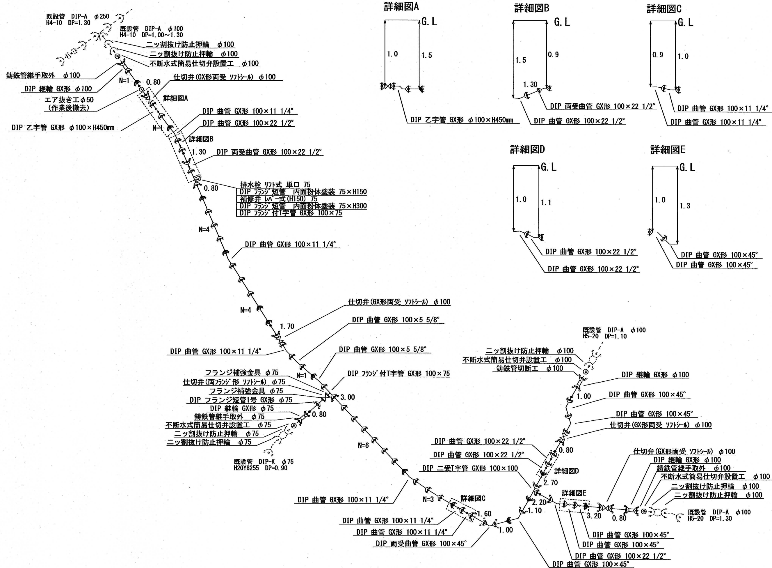
割付図 S=FREE
