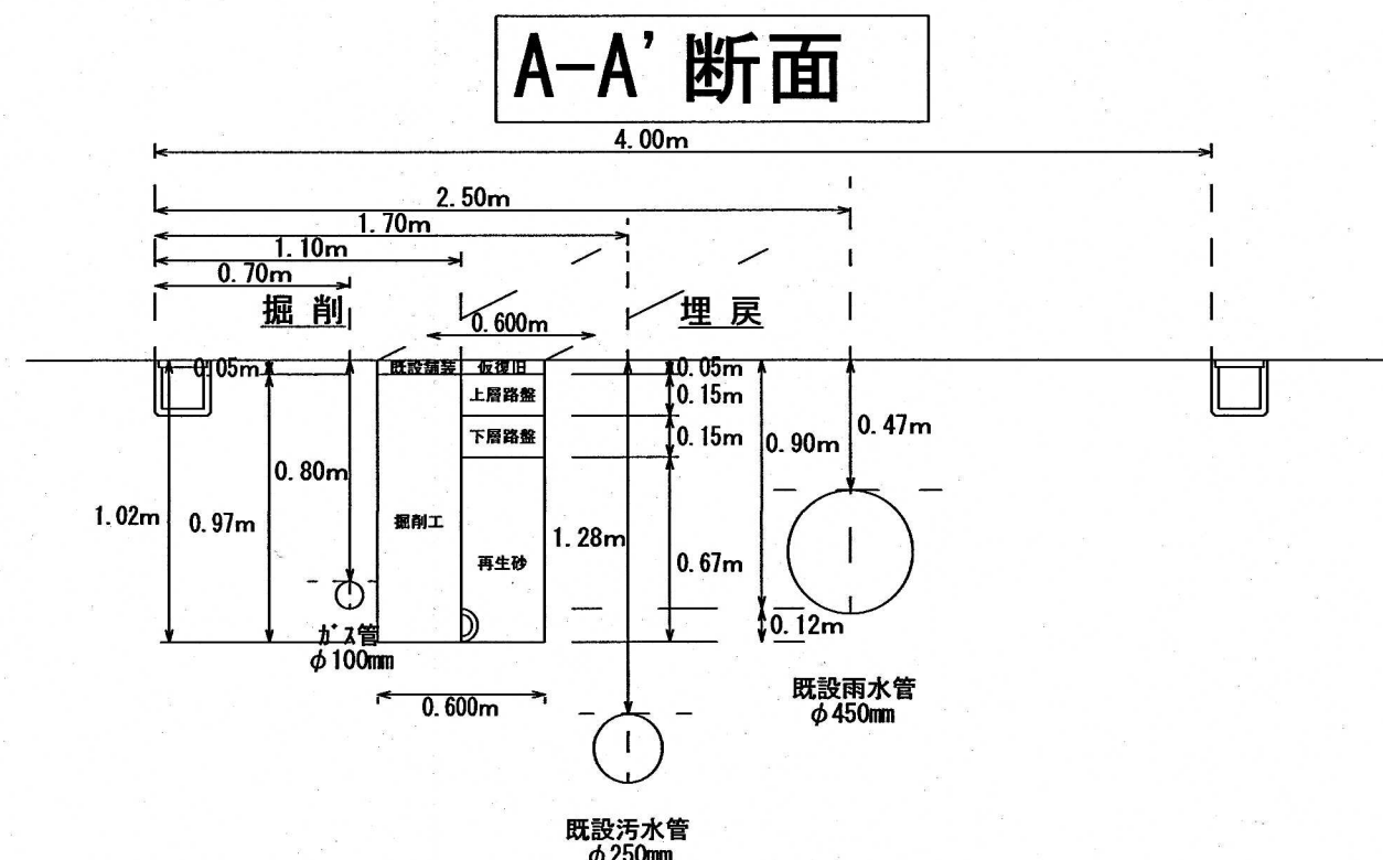
横断面図 S=1/30
