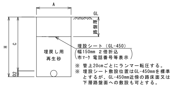
市道（車道）土被掘削表
