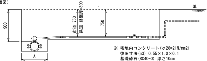
道路止水 (止水栓まで)
