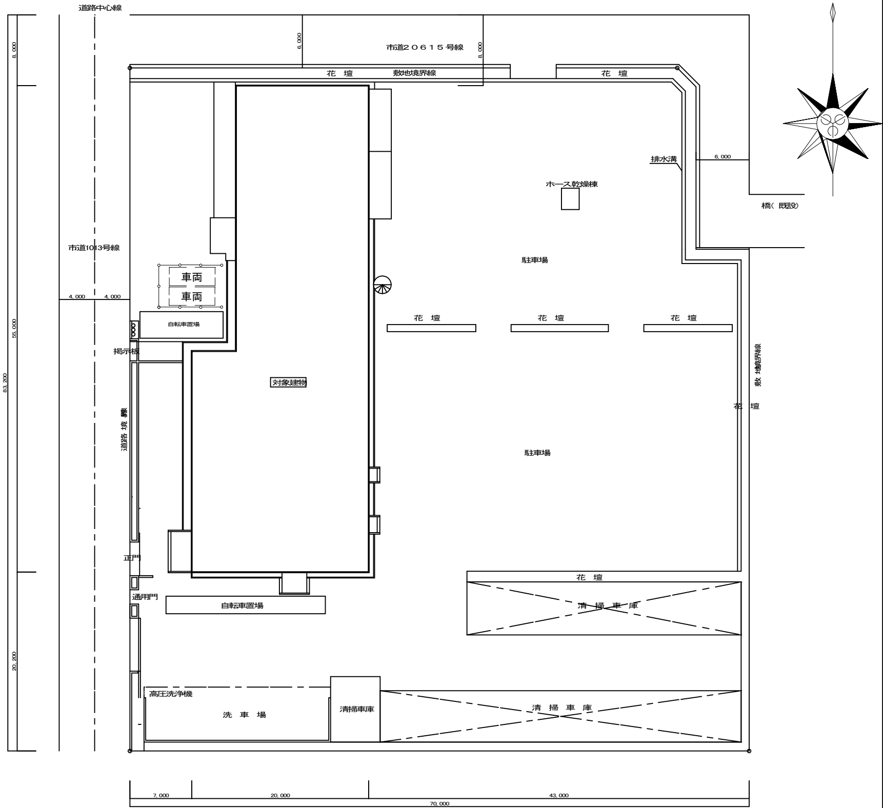
配置図・仮設計画図(参考) S=1/300(A2)
