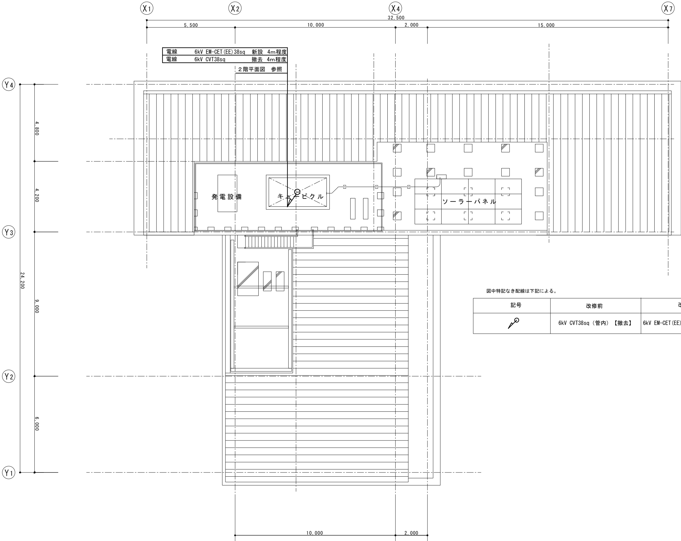
屋上平面図 S=1:100 (A2)
