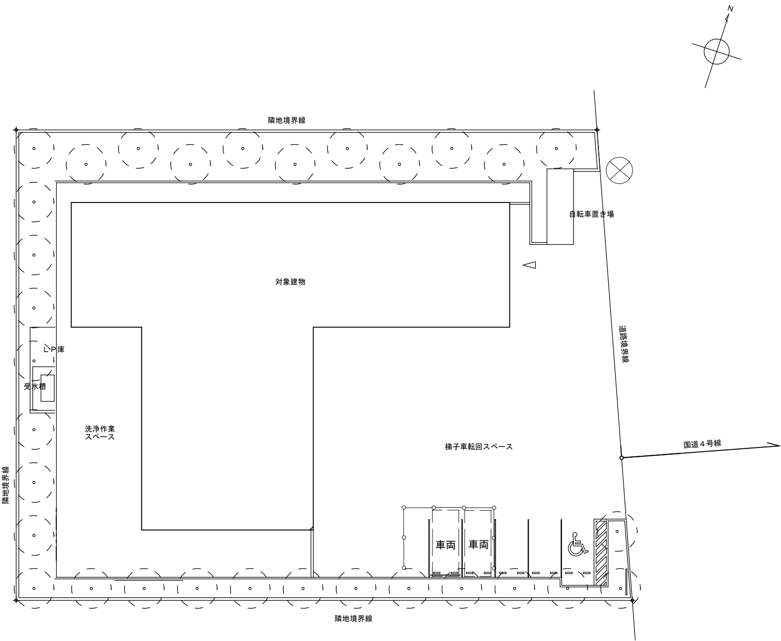
配置図・仮設計画図（参考） S=1/200（A2）
