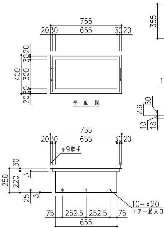
正面図
