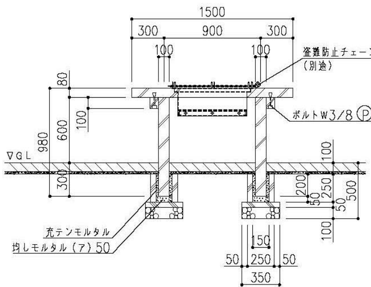
正面図
