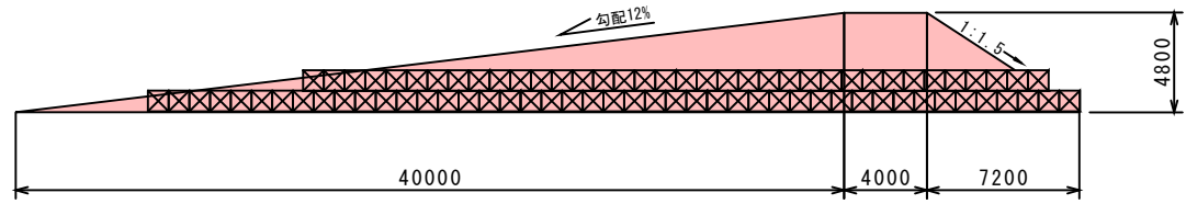
仮設縦断面図 (1 : 200)
