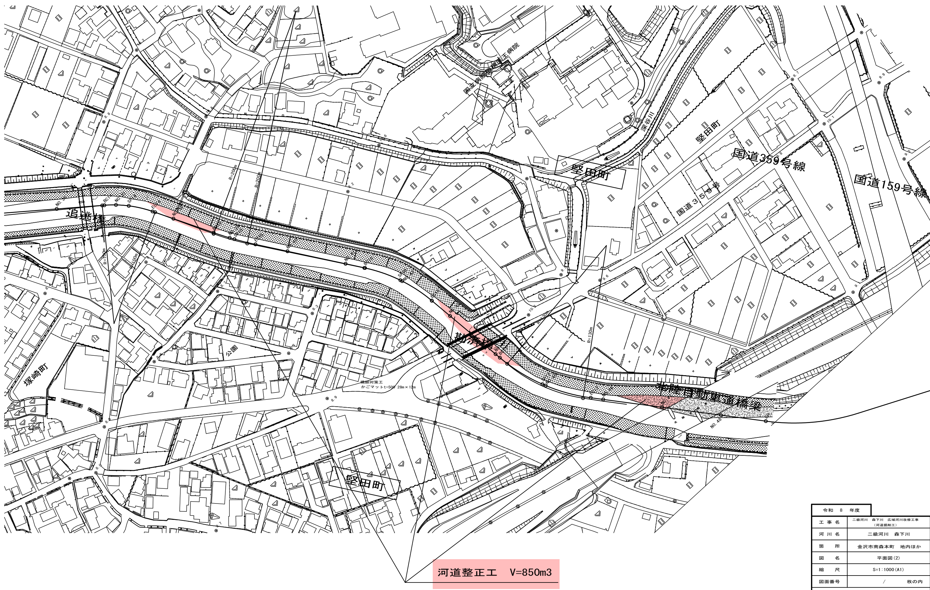
平面図 (2) S=1:1000
