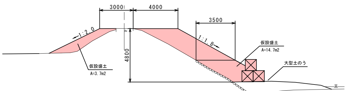
仮設横断面図 (1 : 100)
