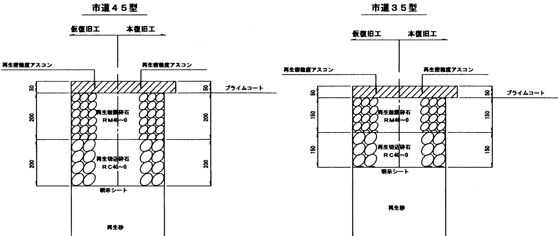
路面復旧組成図 S=FREE
