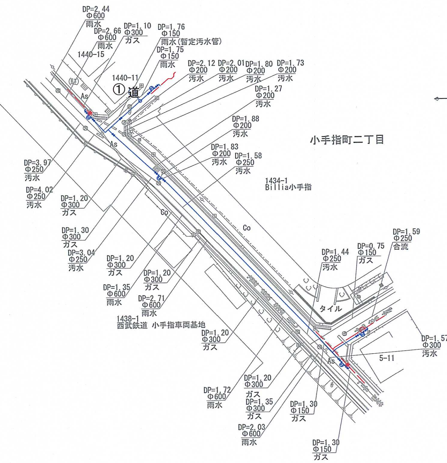
仮設平面図 1/500
