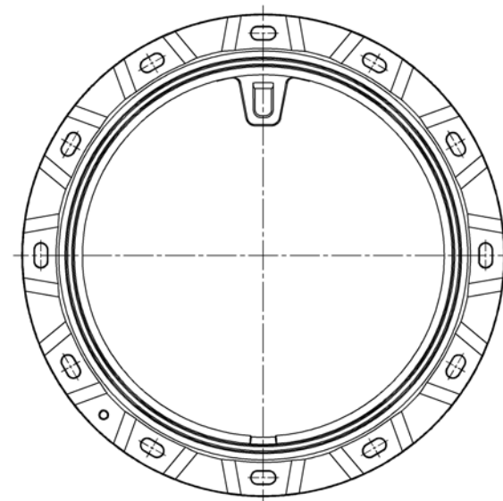
受枠平面図
