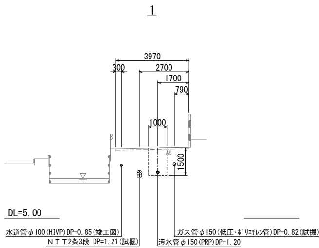
横断面図 縮尺 1:100
