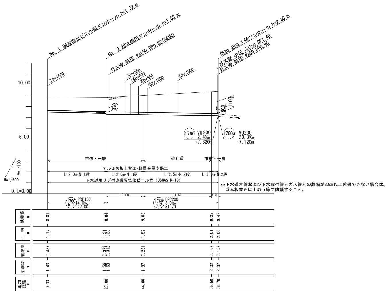
縦断面図 縮尺 縦1:100 横1:500
