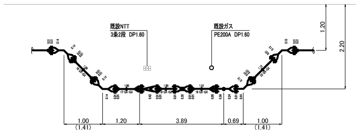
① ② 詳細図
