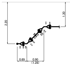
③ ④ 詳細図
