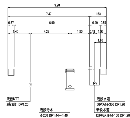
④断面
