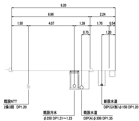
②断面
