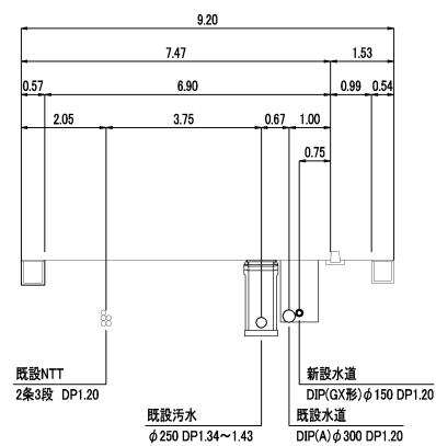
③断面
