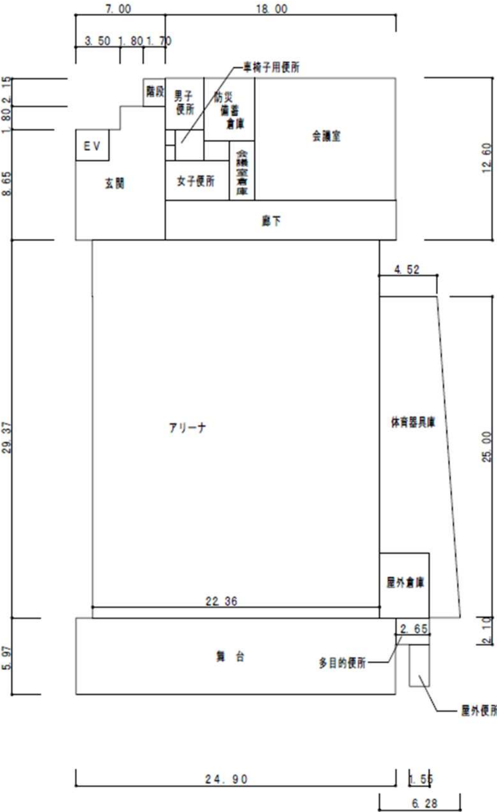
1 階平面図
