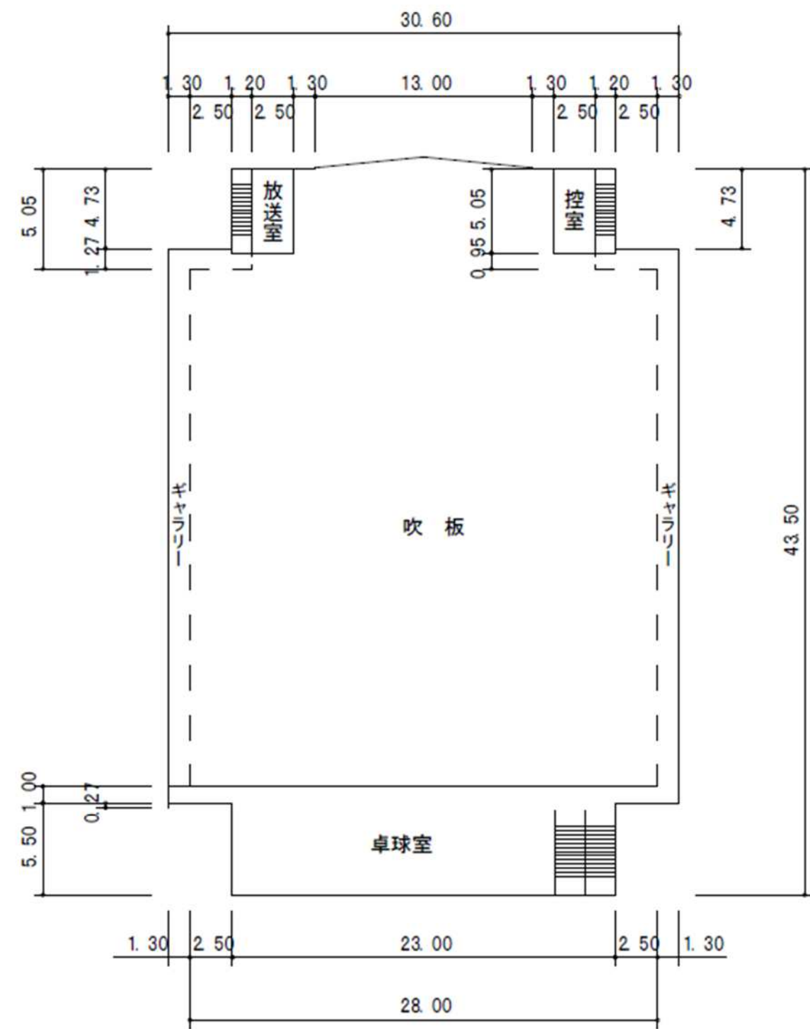
③ 2階
