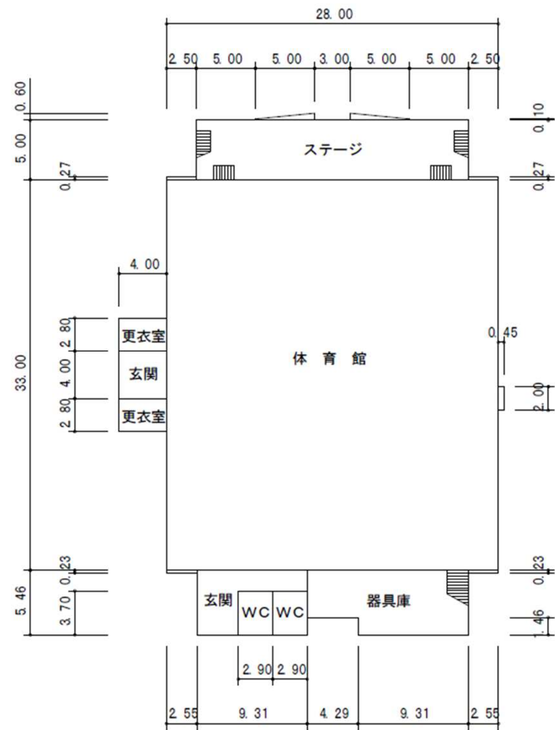
③ 1階
