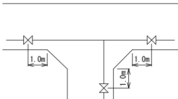
仕切弁位置図
