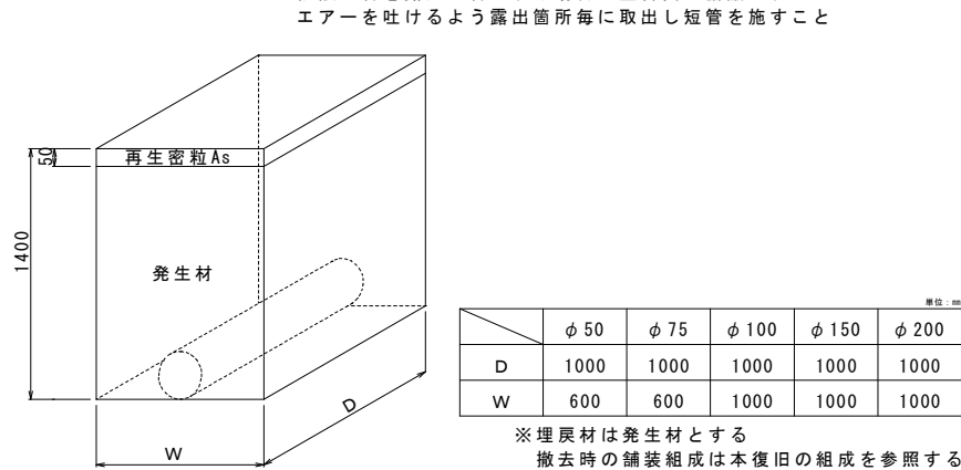
⑤ 取出し土工標準図
