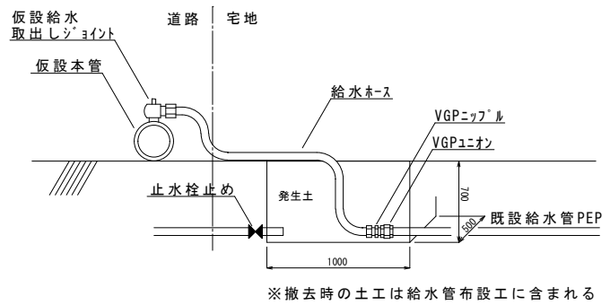
② 宅地内接続
