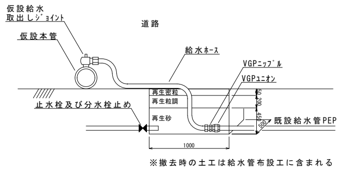
③ 道路接続
