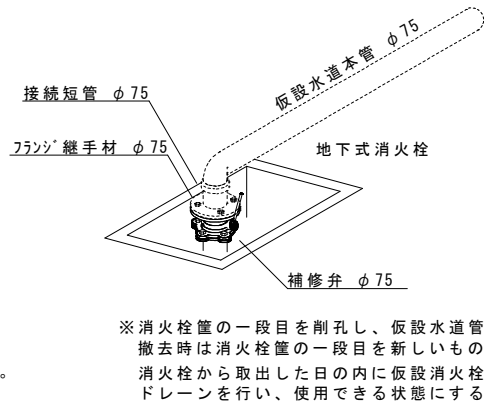
④ φ75（地下式消火栓からの取出し）
