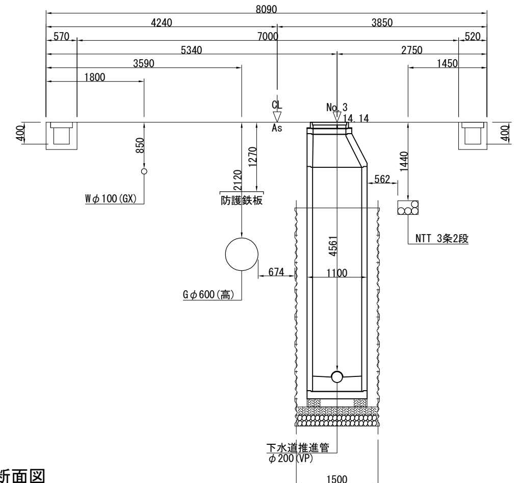
No. 3 断面図
