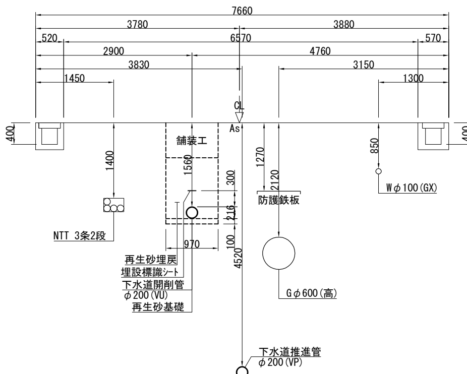
②—②断面図
