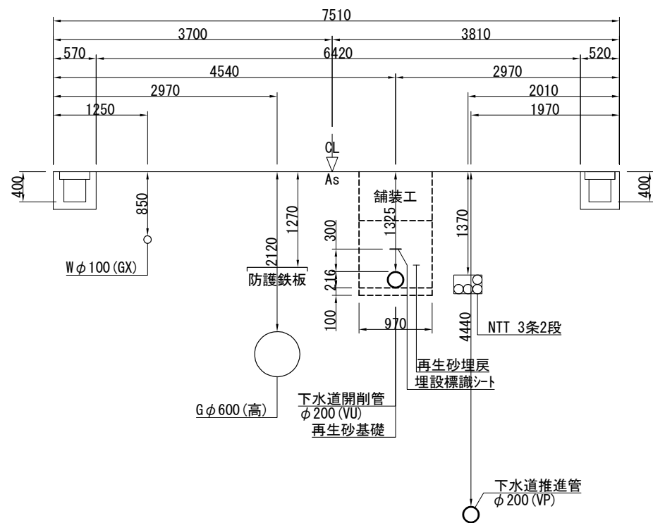
①—①断面図
