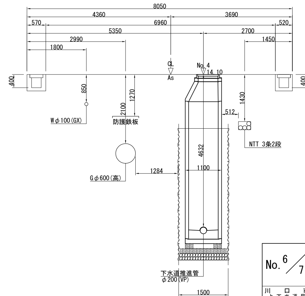
No. 4 断面図
