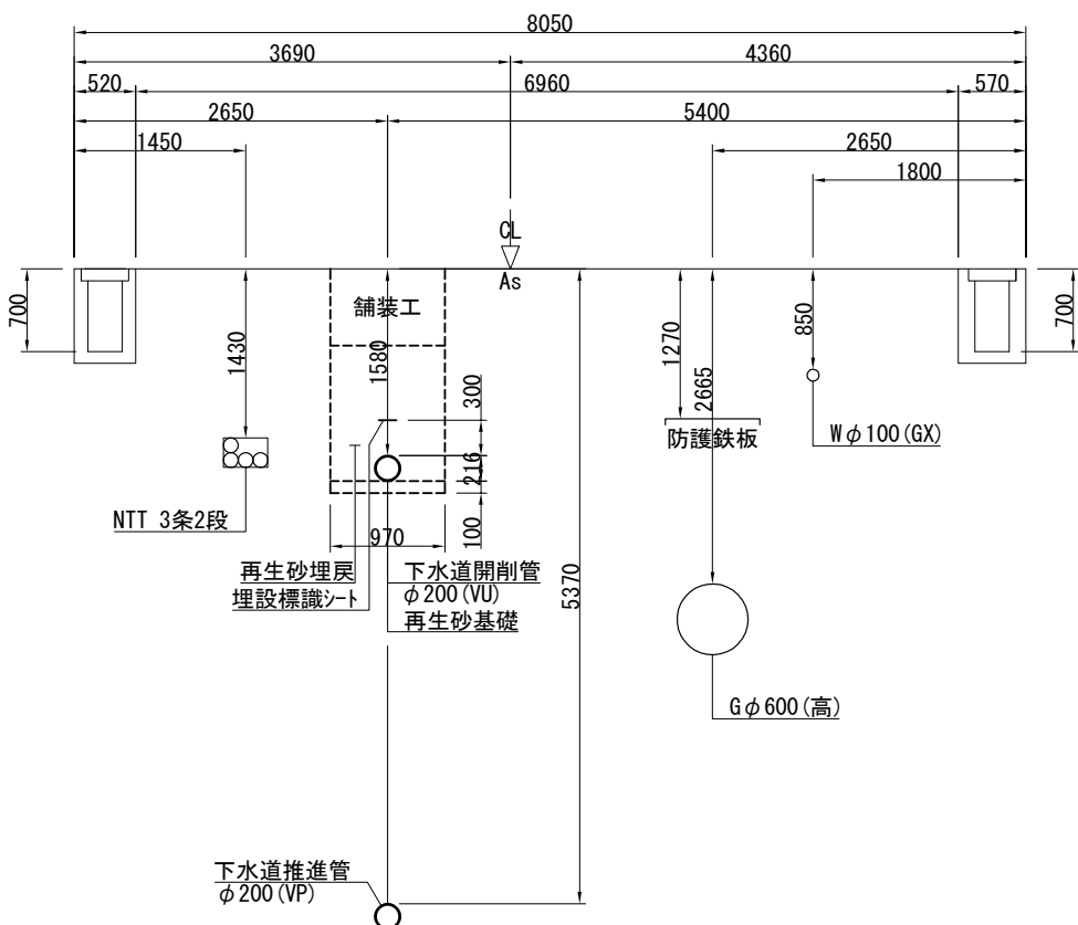
⑤—⑤断面図
