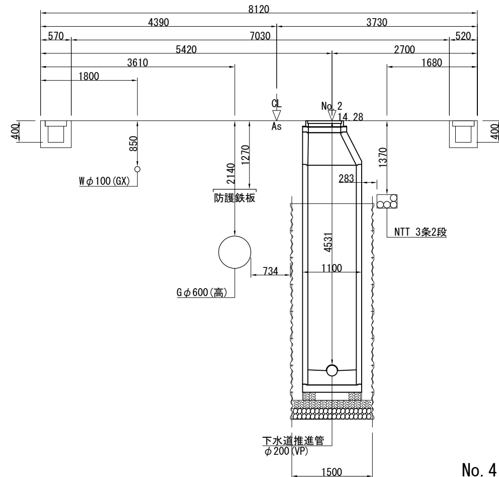
No. 2 断面図
