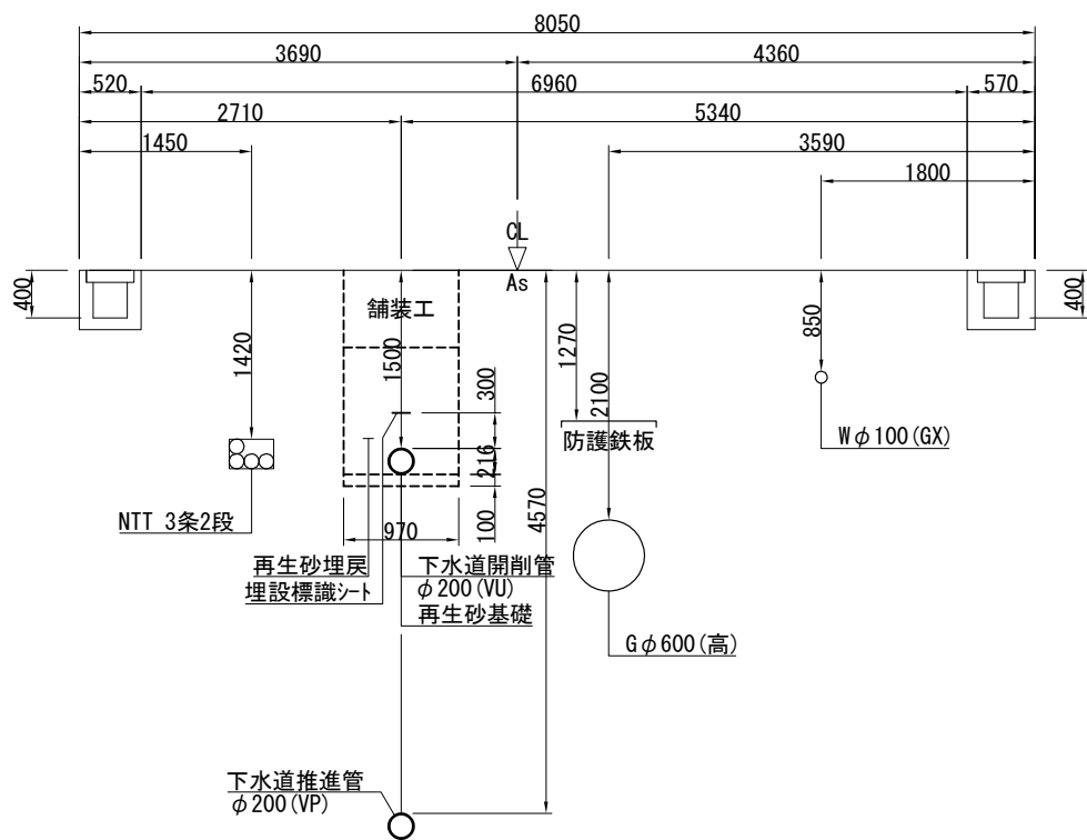
④—④断面図
