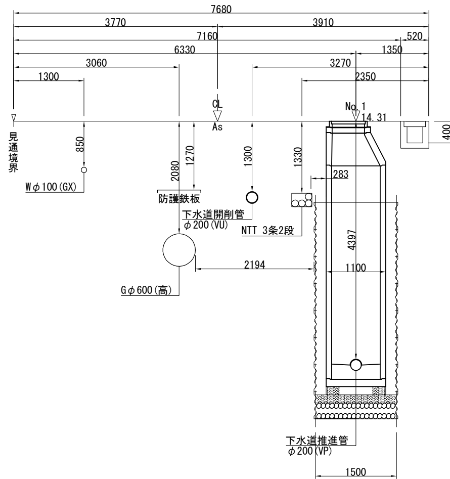
No. 1 断面図
