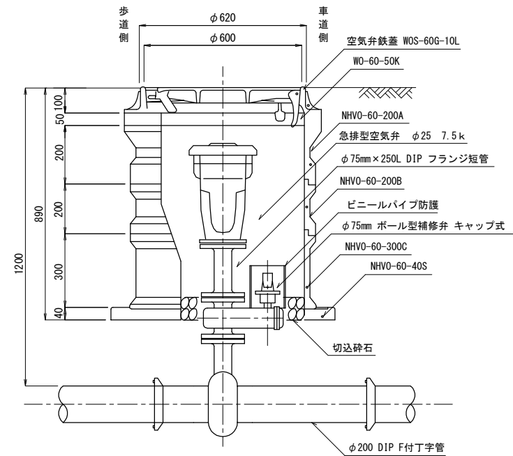
断面図
