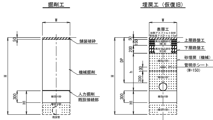
町道（車道一層）
