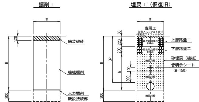
町道（車道二層）
