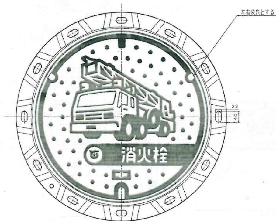
蓋，受栓平面図
